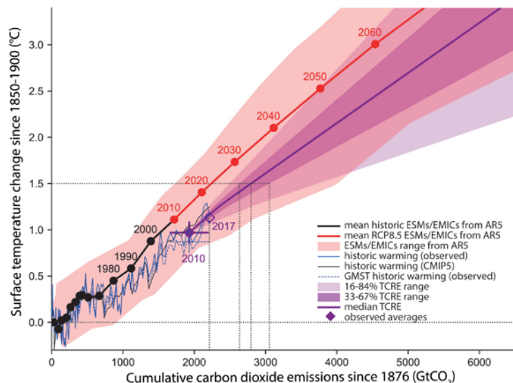
Abb. 6: Aus dem IPCC Report SR15
